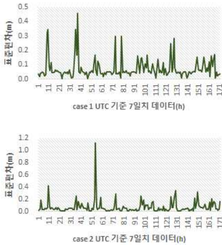
그림 4. 표준편차 비교
